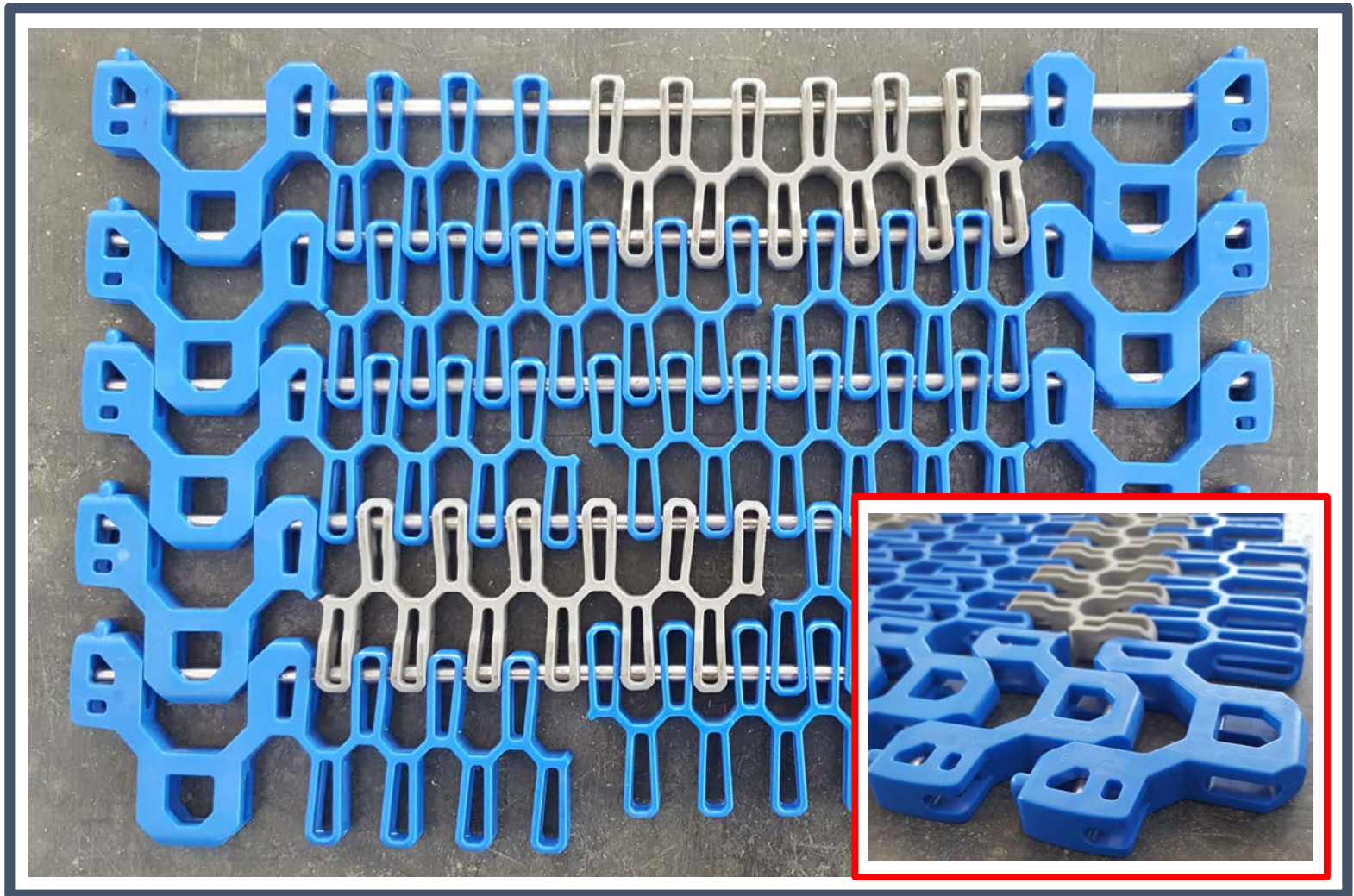
Nastro PLASTICA con rete passo LARGO Con inserti di gomma antiscivolo
