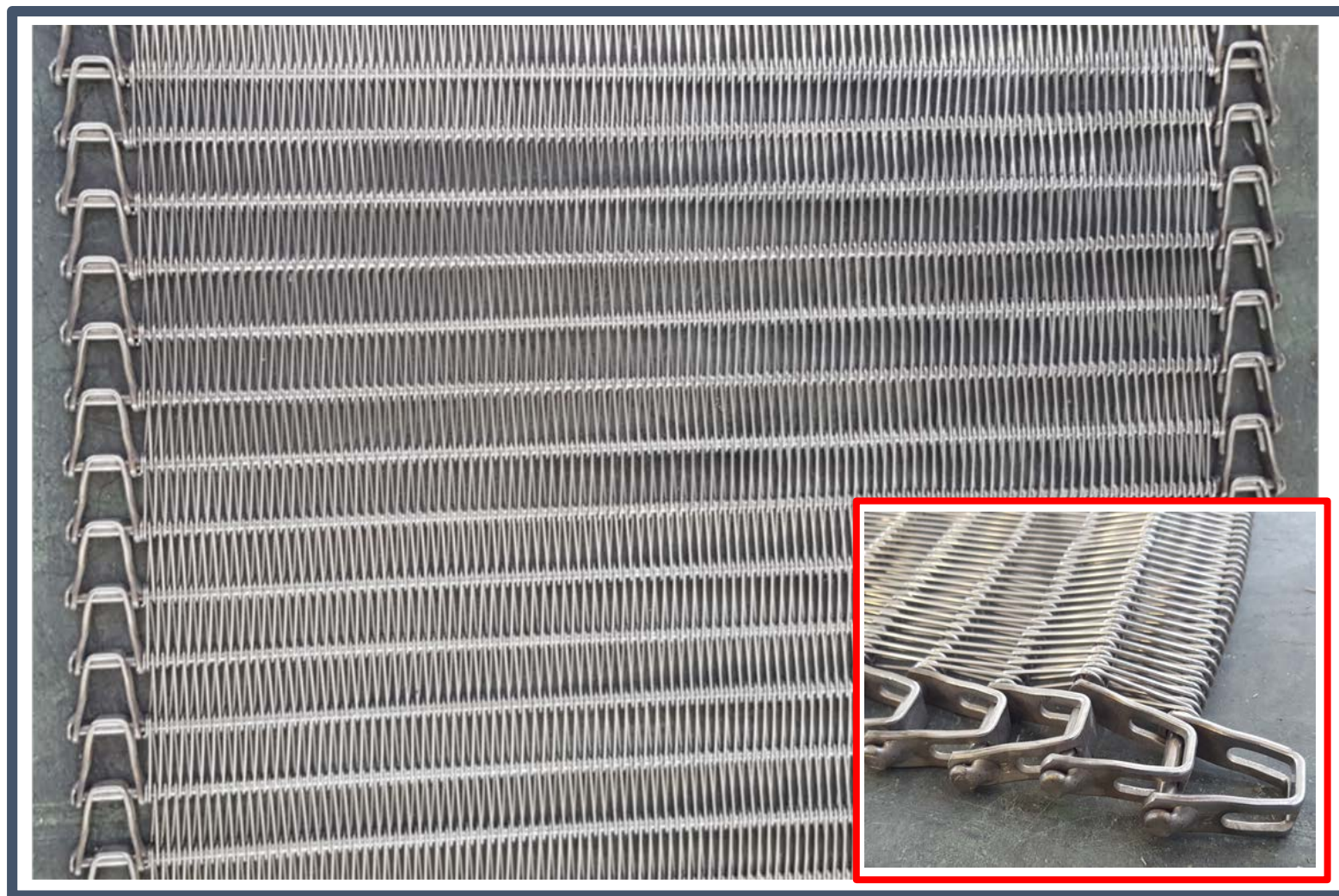
Nastro INOX passo STRETTO 8mm Senza alette laterali
