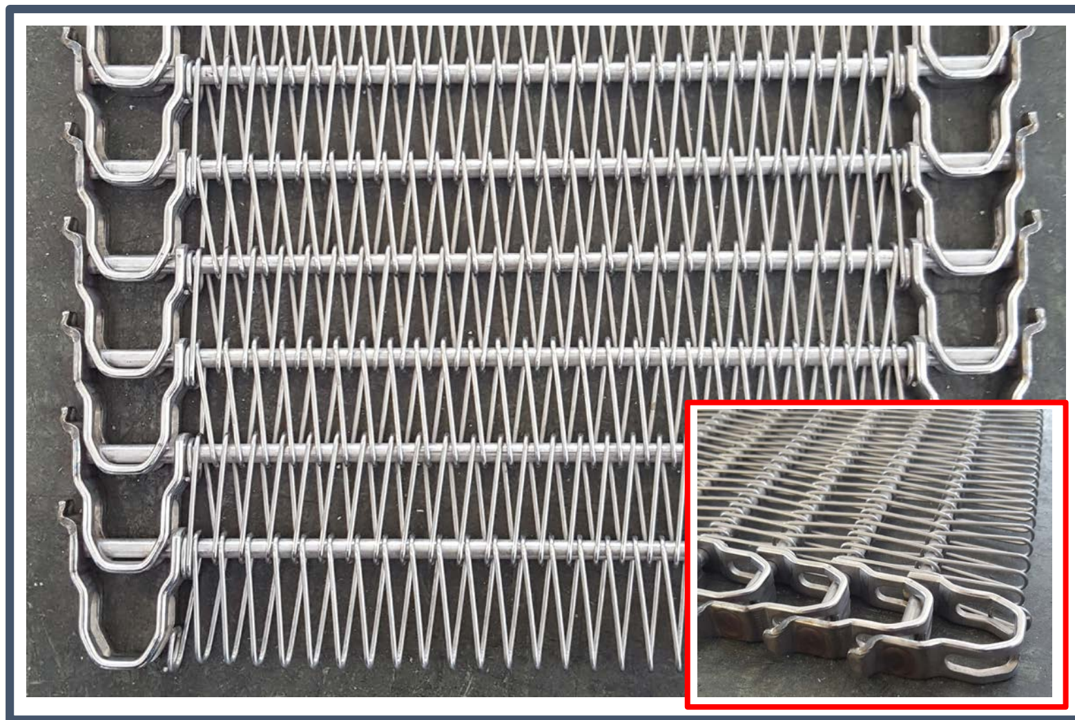
Nastro INOX passo LARGO 12mm Senza alette laterali
