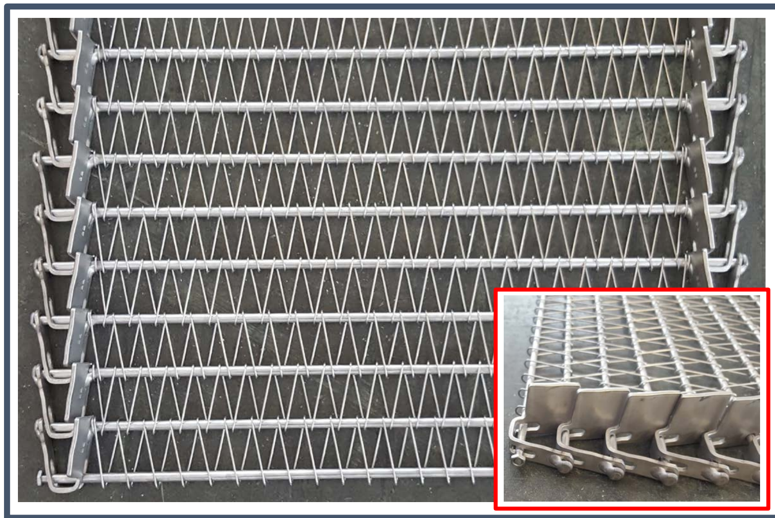
Nastro INOX passo LARGO 18mm Con alette laterali alte
