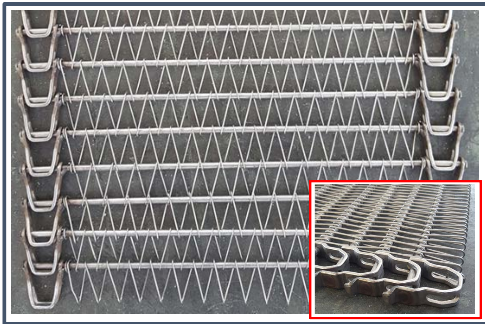
Nastro INOX passo LARGO 18mm Senza alette laterali
